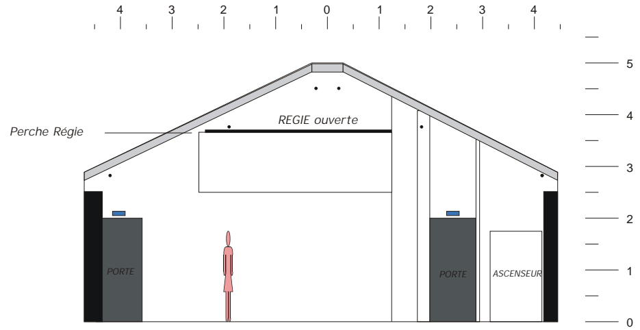
COUPE TRANSVERSALE (Vue du Lointain)
