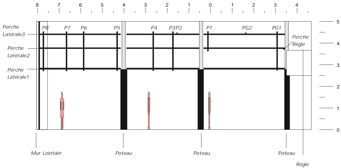
COUPE LONGITUDINALE
